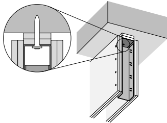
Mocowanie głowicy odchylającej za pomocą pasków gipsowych (opcjonalnie z uszczelniaczem)
