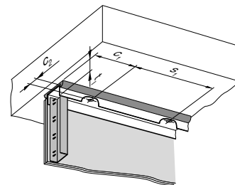
Mocowanie szyny połączenia przesuwnej (opcjonalnie z uszczelniaczem)
