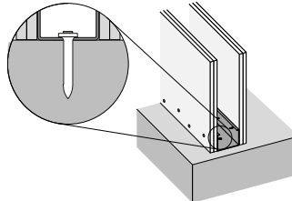
Fissaggio guida fissa
