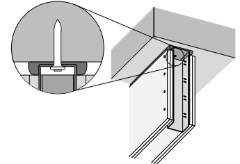
Fissaggio del binario della testa di deviazione (in via opzionale con sigillante)
