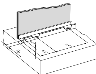
Fissaggio guida fissa
