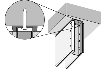
Mocowanie szyny połączenia przesuwnej (opcjonalnie z uszczelniaczem)
