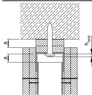
Fijación del cabezal de desvío con tiras de yeso (opcional con sellador)
