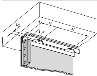
Umlenkkopfbefestigung mit Gipsstreifen (optional mit Dichtmasse)
