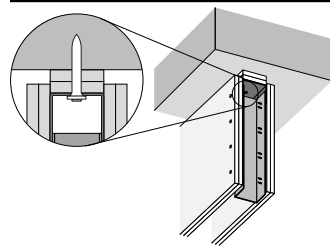
Fixation à tête de déflexion avec bandes de plâtre (en option avec matériau d'étanchéité)
