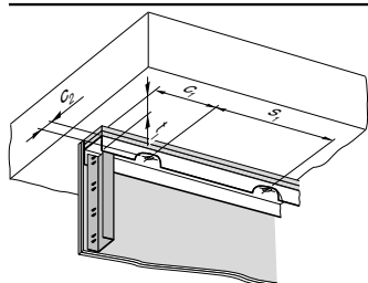
Mocowanie głowicy odchylającej za pomocą pasków gipsowych (opcjonalnie z uszczelniaczem)
