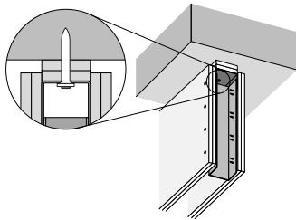
Fissaggio della testa di deviazione con strisce di gesso (opzionale con sigillante)
