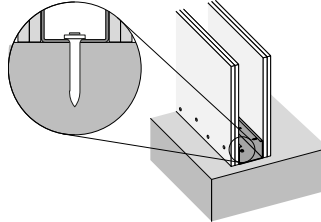
Stałe mocowanie profilu
